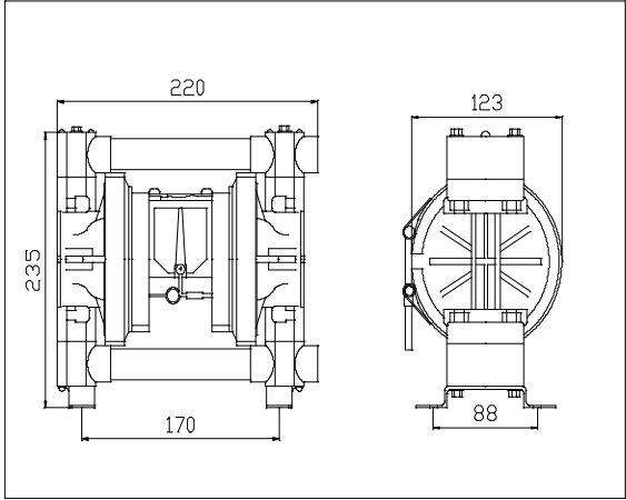
安装尺寸图 单位:mm
