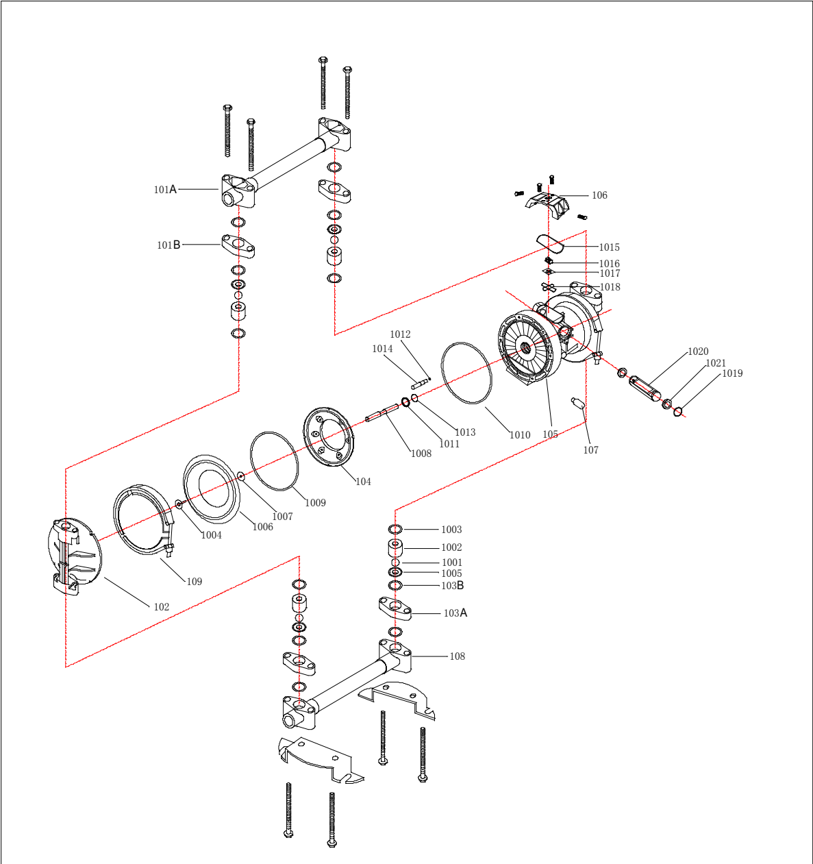
零部件明细表 Parts List
