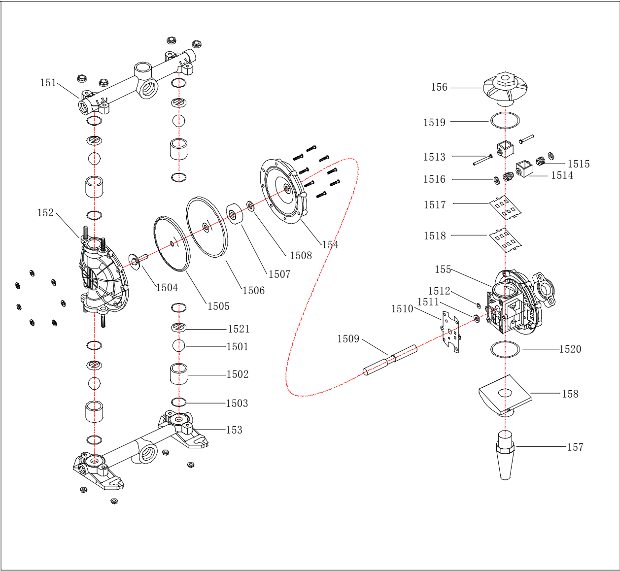
零部件明细表 Parts List
