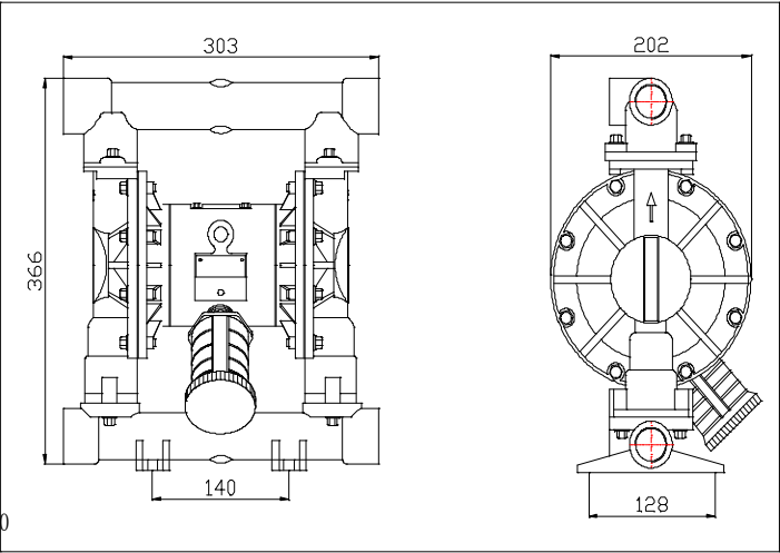
安装尺寸图
