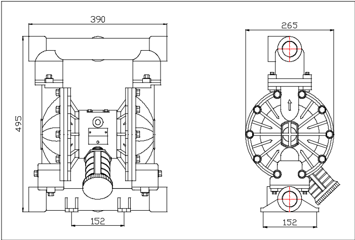
安装尺寸图
