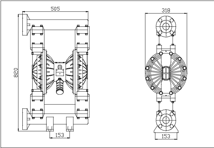
安装尺寸图
