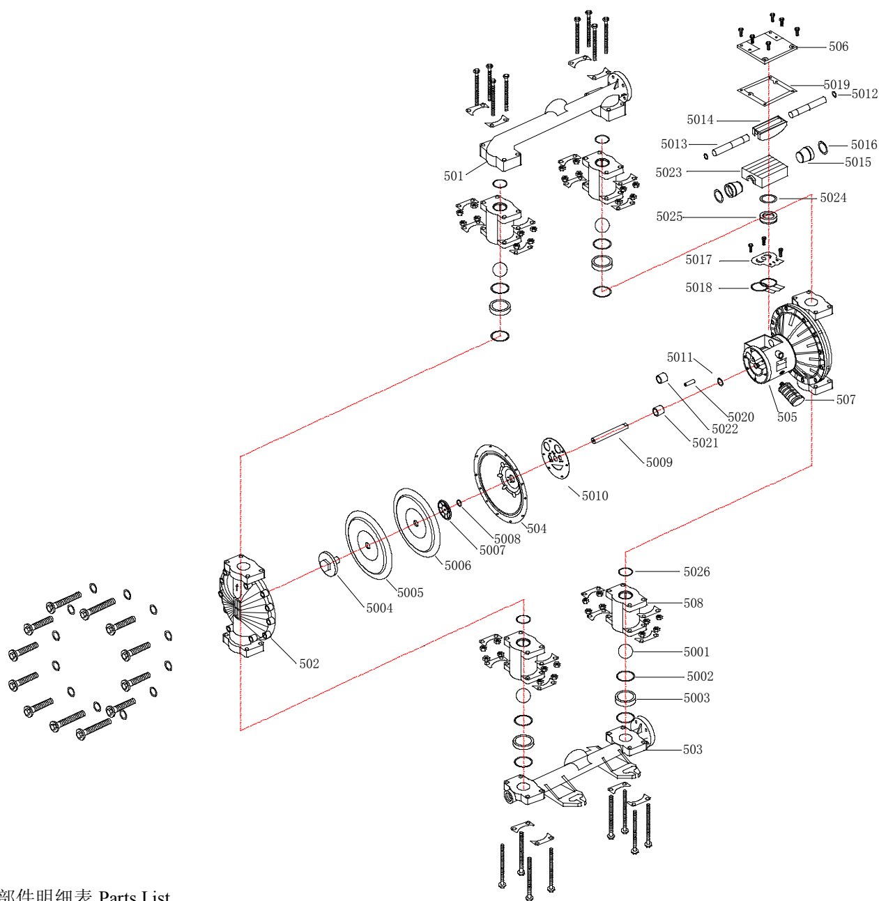
零部件明细表 Parts List
