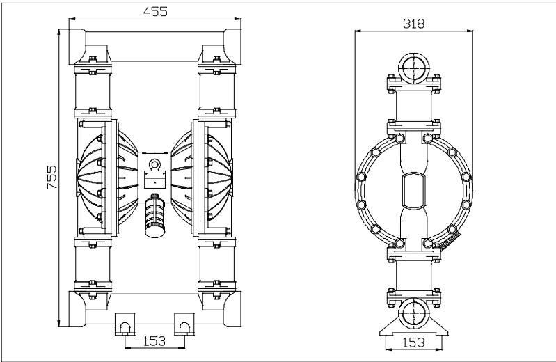
安装尺寸图
