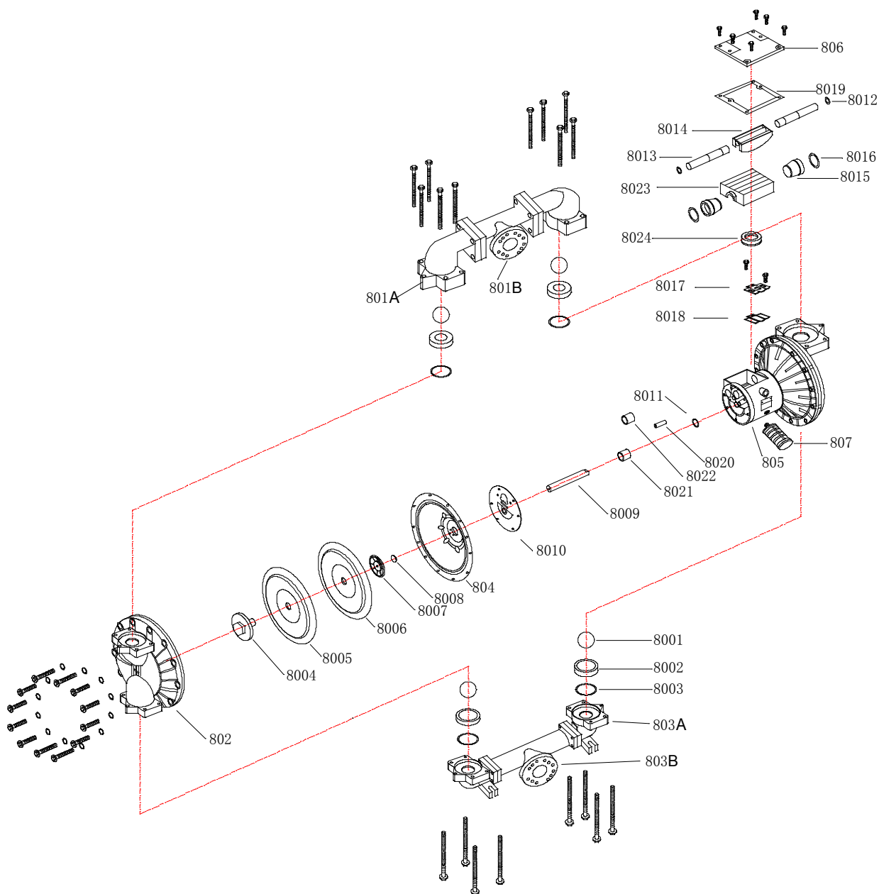
零部件明细表 Parts List
