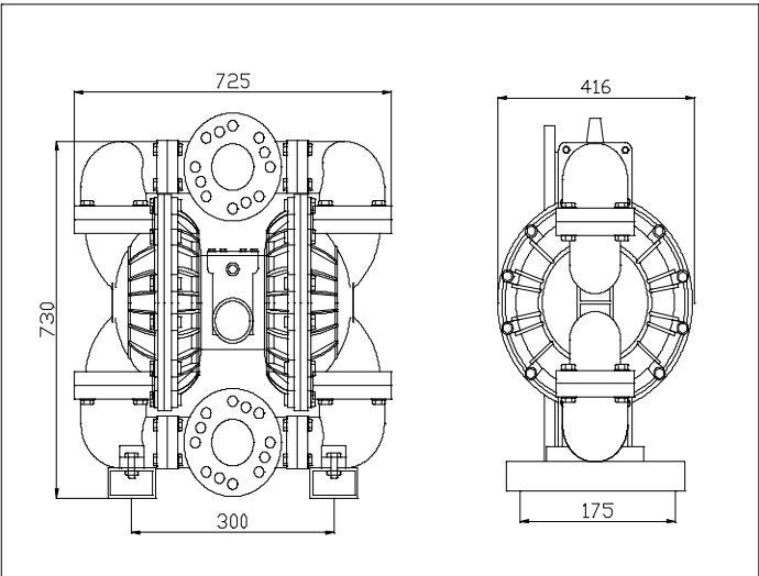
安装尺寸图
