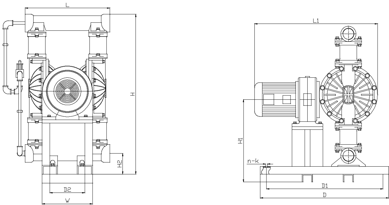
安装尺寸图
