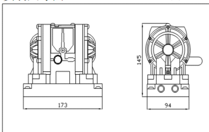
安装尺寸图
